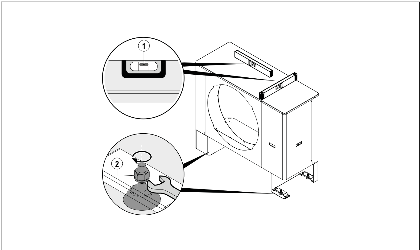
FIG. 39 (Livellamento della macchina)
