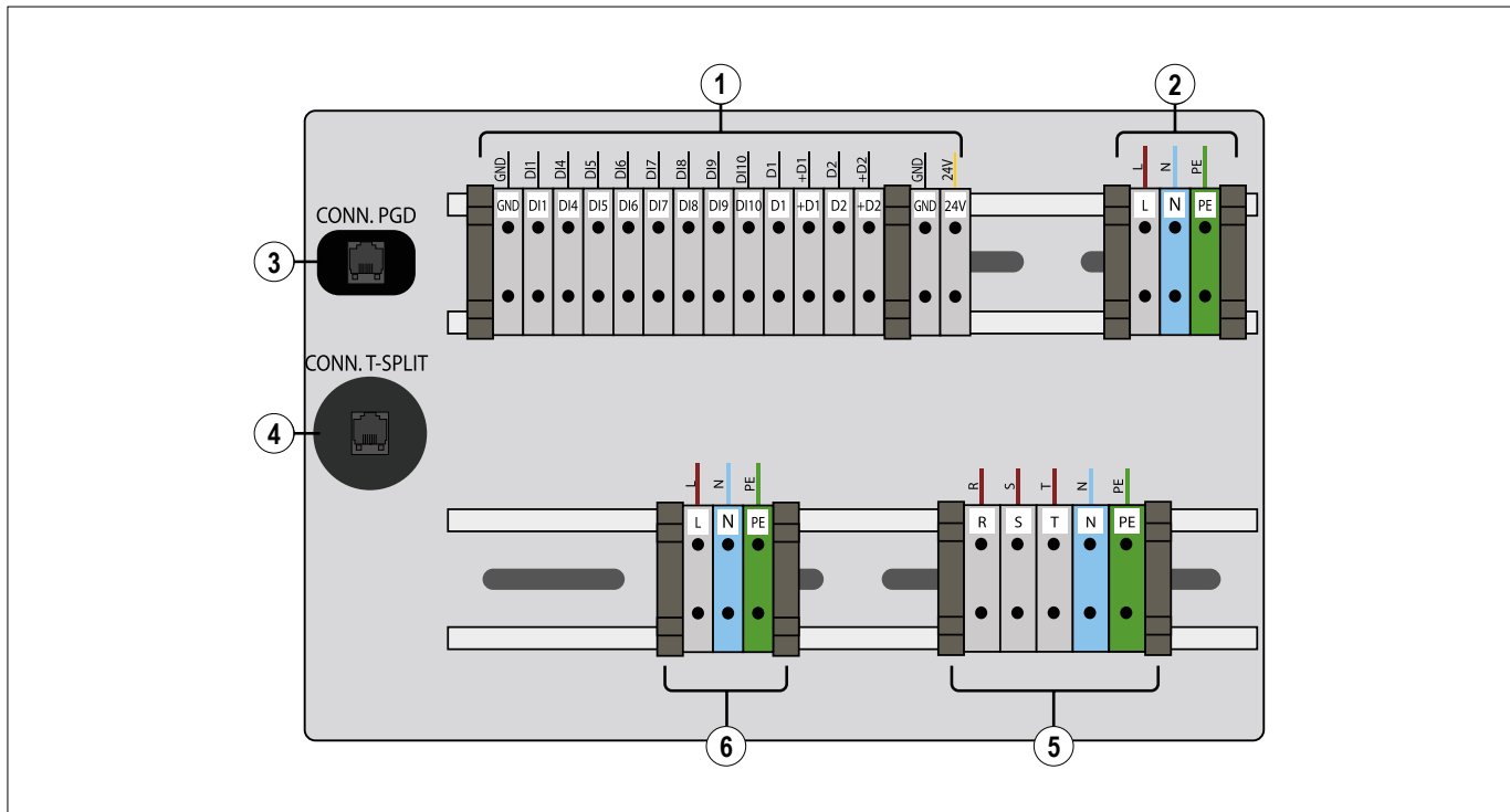
FIG. 51 (Morsetti quadro elettrico secondario per PDC doppia alimentazione)
