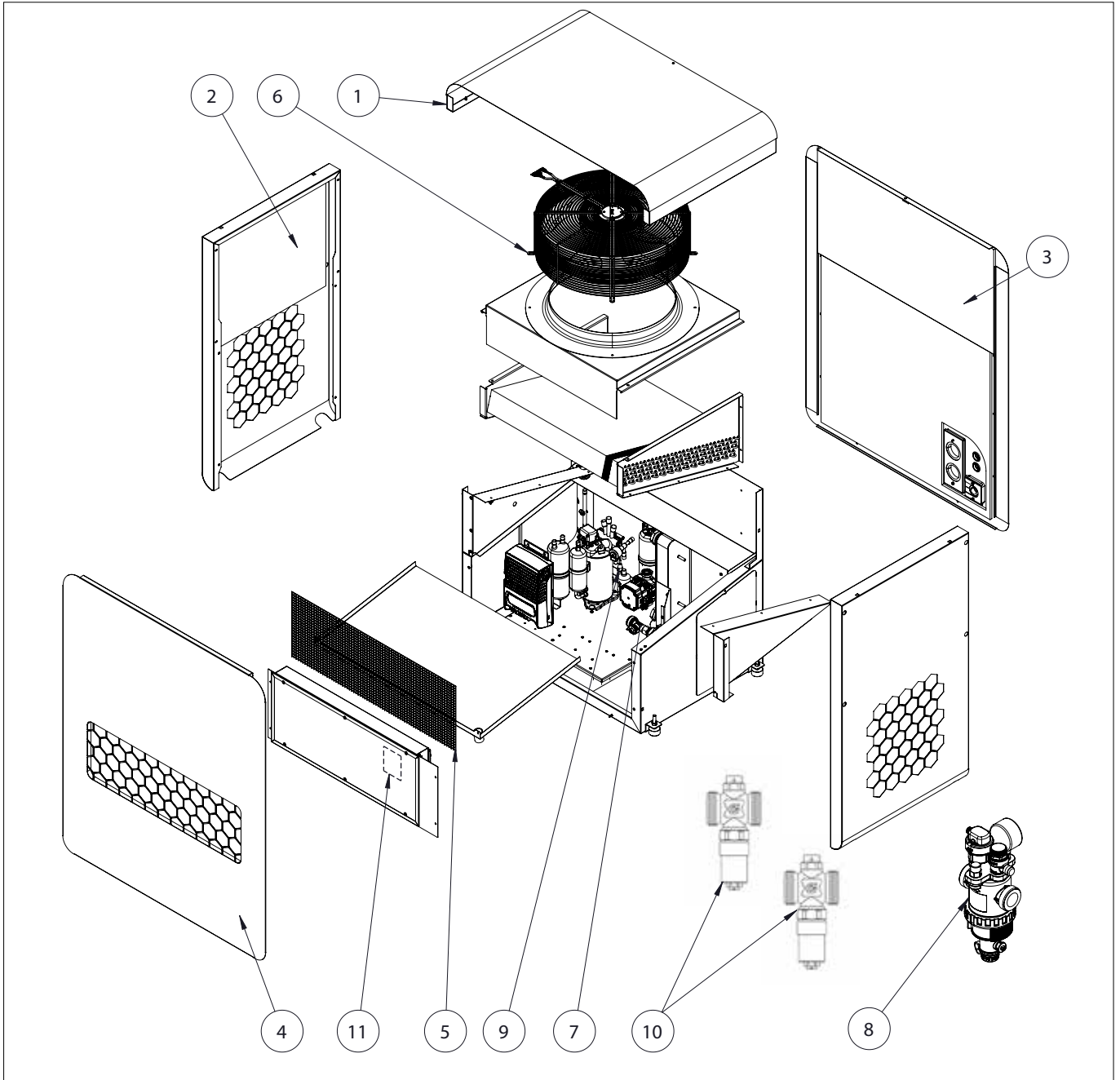
FIG. 29 (Ripari e dispositivi di protezione XS versione Alta e Bassa)
