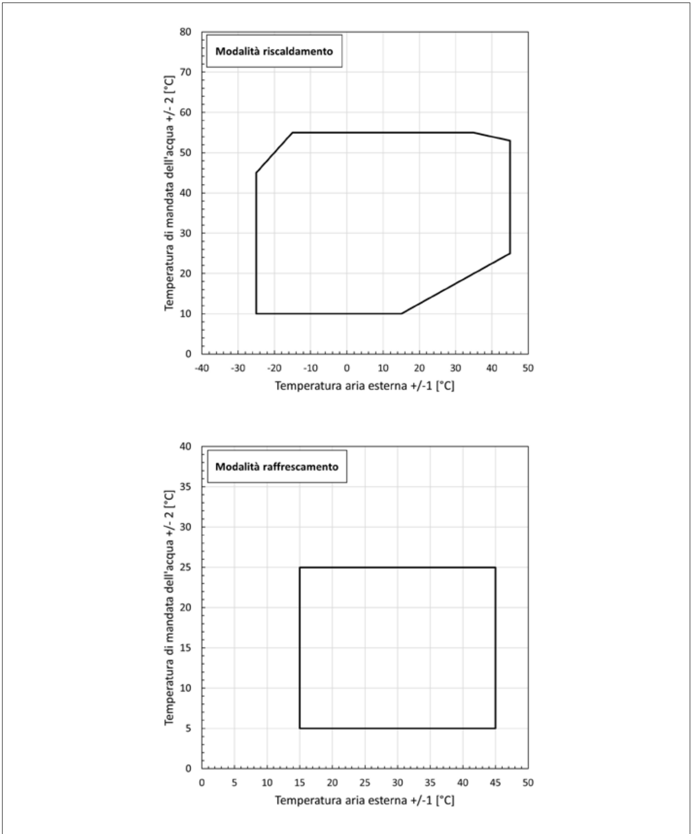
FIG. 9 (Modalità di riscaldamento e raffreddamento Serie LR - LR Plus)
