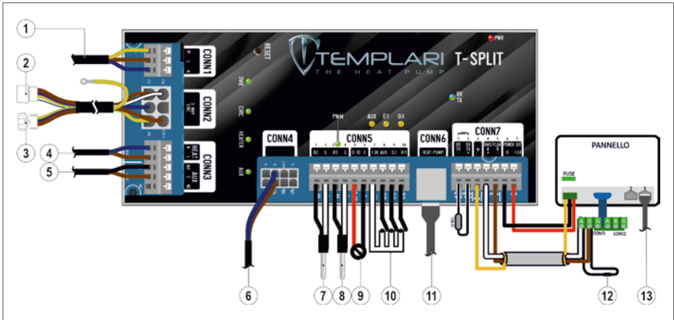
FIG. 61 (Modulo T-Split)
