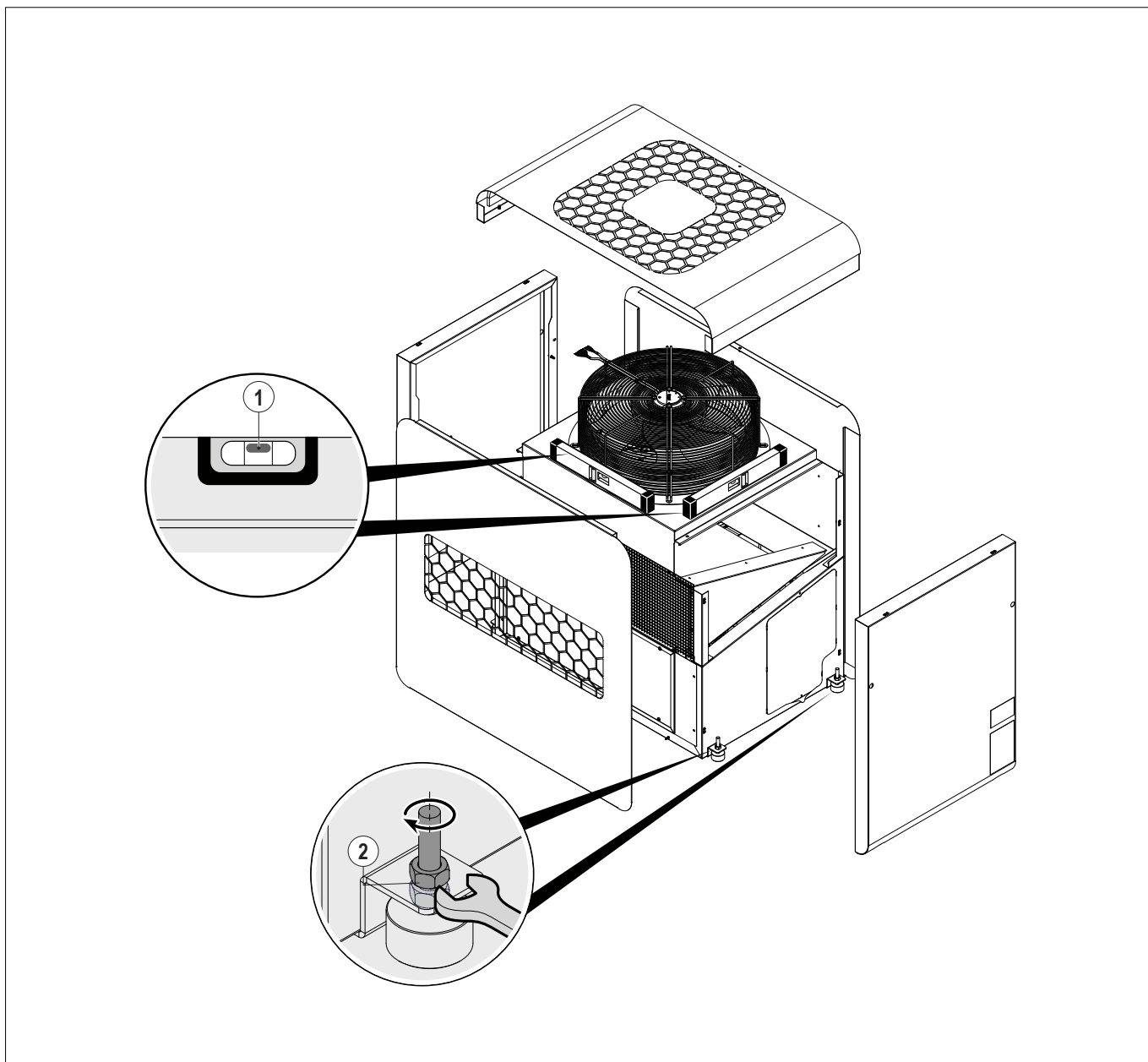
FIG. 40 (Livellamento della macchina)
