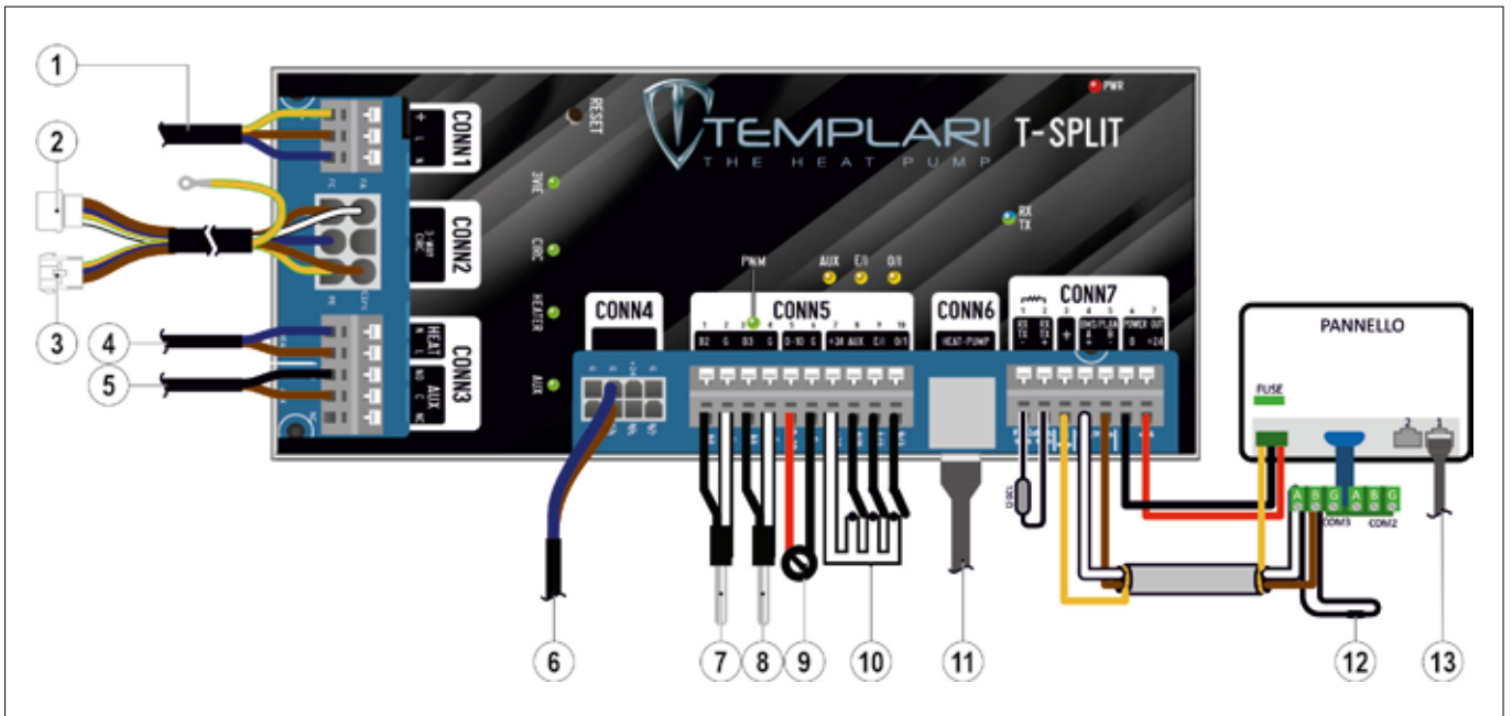
FIG. 52 (Modulo T-Split)
