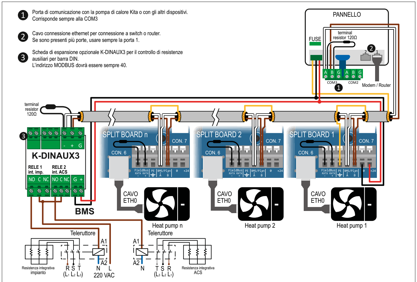
FIG. 57 (Connessione elettrica Multi-KITA)
