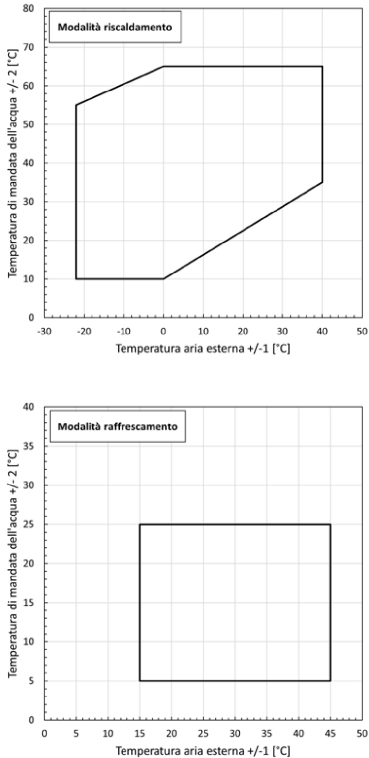
FIG. 7 (Modalità di riscaldamento e raffrescamento Serie MP - LP)
