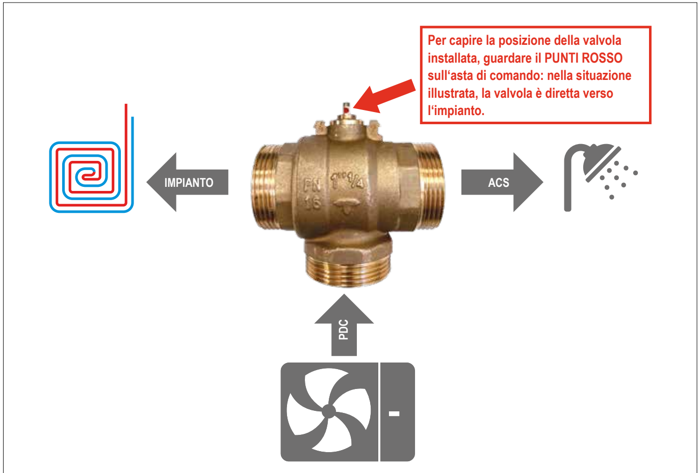
FIG. 55 (Collegamenti idraulici valvola a tre vie)
