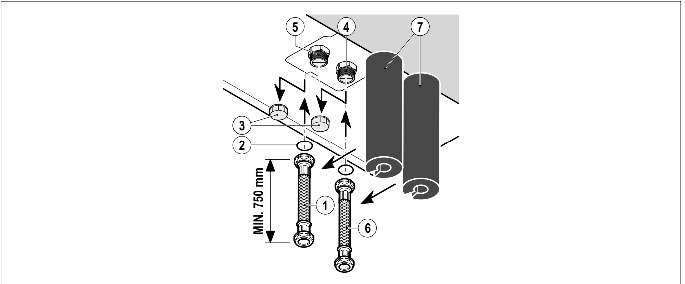
FIG. 41 (Collegamento alla fonte di energia idrica)
