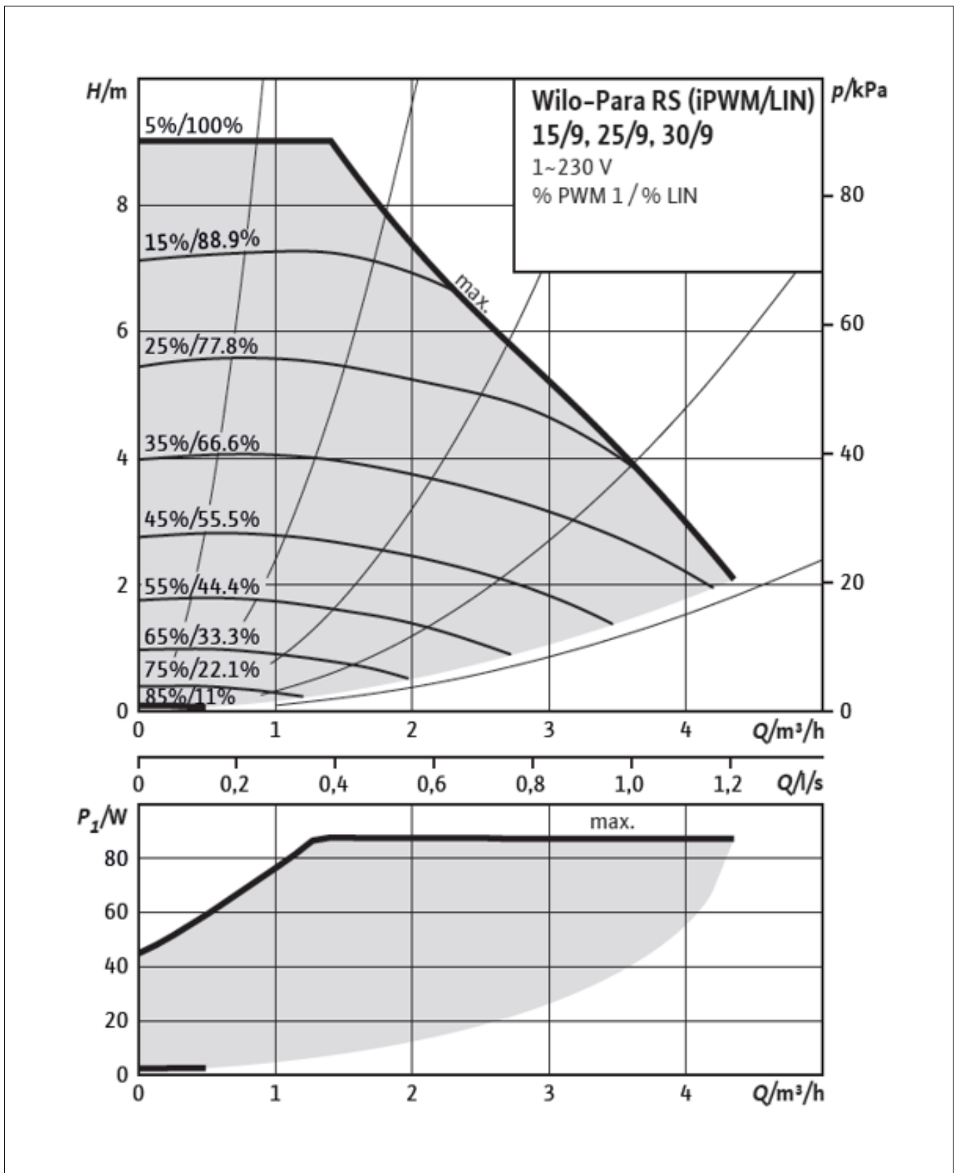
FIG. 13 (Curve e caratteristiche circolatore tipo Wilo Para 25/9 e Wilo Para R 25/9)
