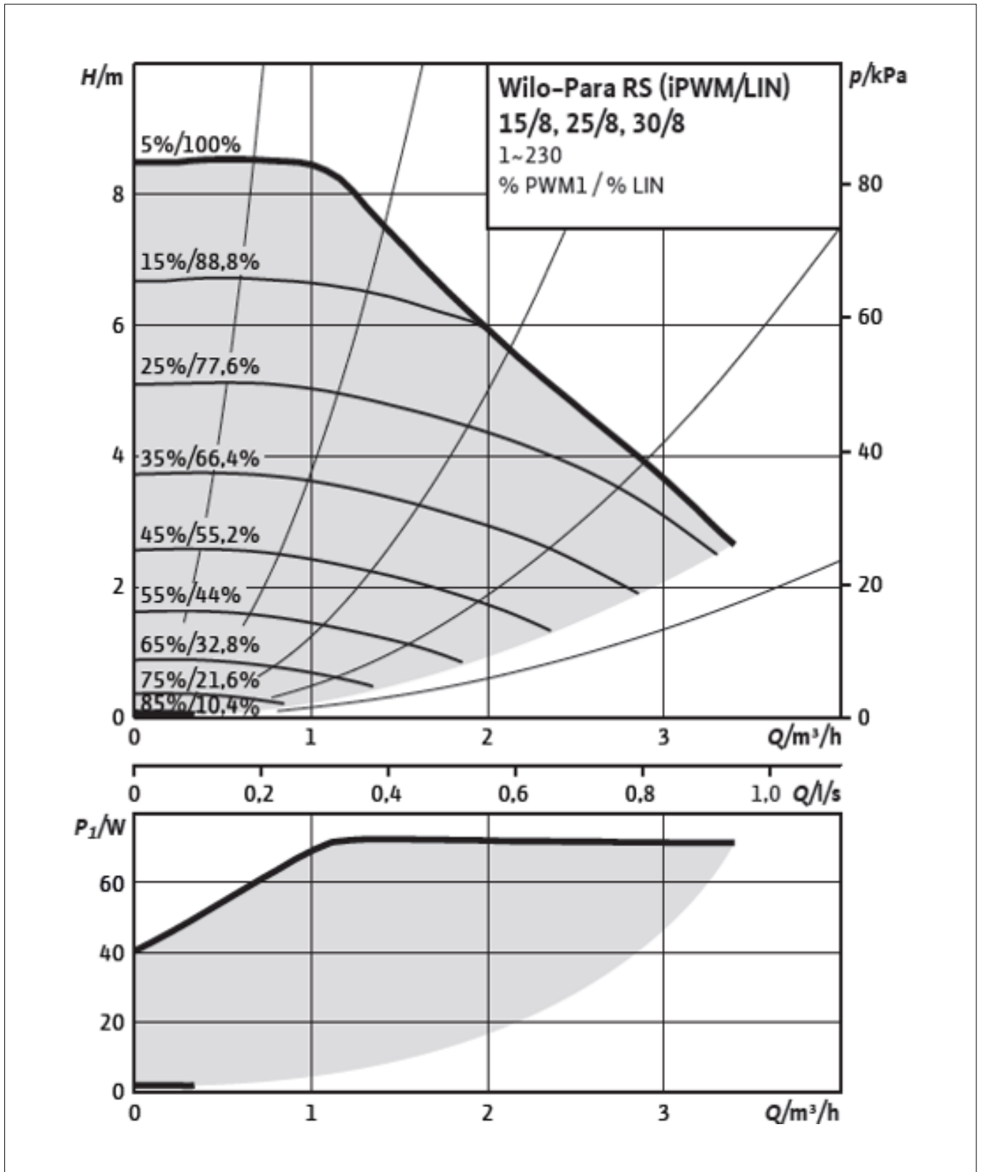
FIG. 11 (Curve e caratteristiche circolatore tipo Wilo Para 25/8 e Wilo Para R 25/8)
