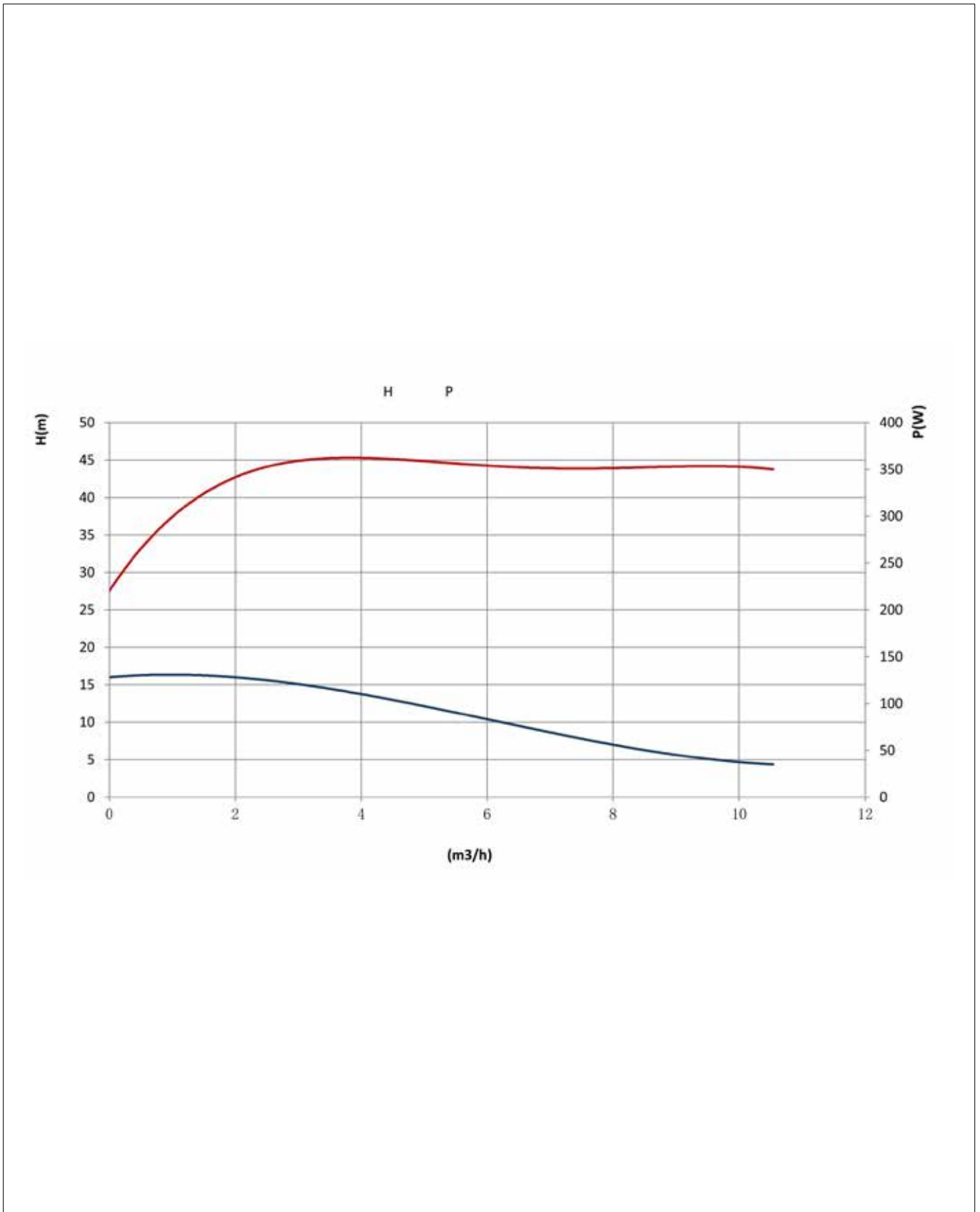
FIG. 15 (Curve e caratteristiche circolatore tipo Templari Gra 32-17 H Pro/180)
