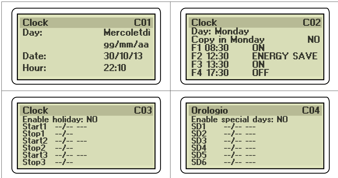
FIG. 74 (Menù Orologio/fasce)
