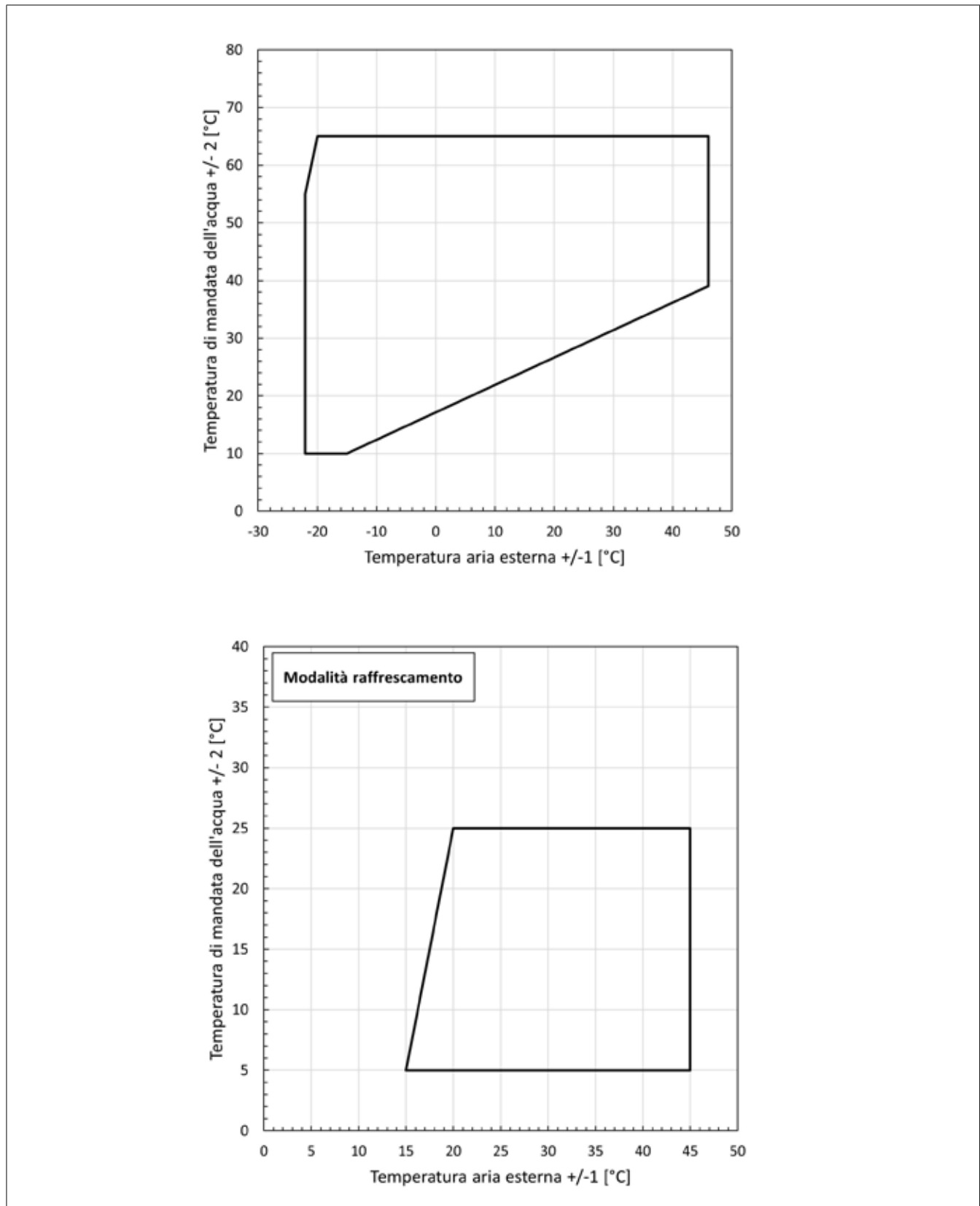
FIG. 10 (Modalità di riscaldamento e raffreddamento Serie XS - S)
