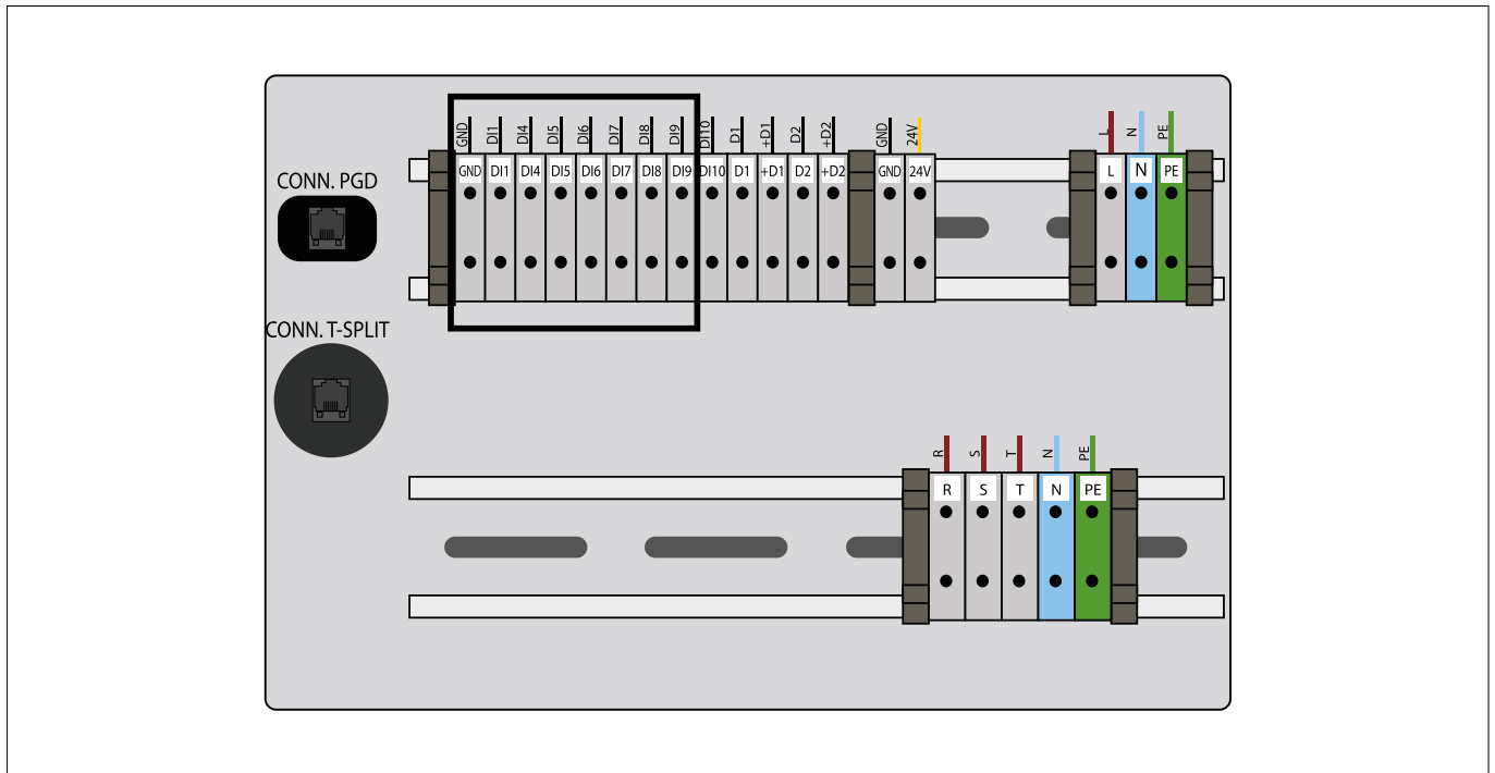
FIG. 64 (Connessione elettrica DI9-GND in caso di connessione bus su P-LAN)
