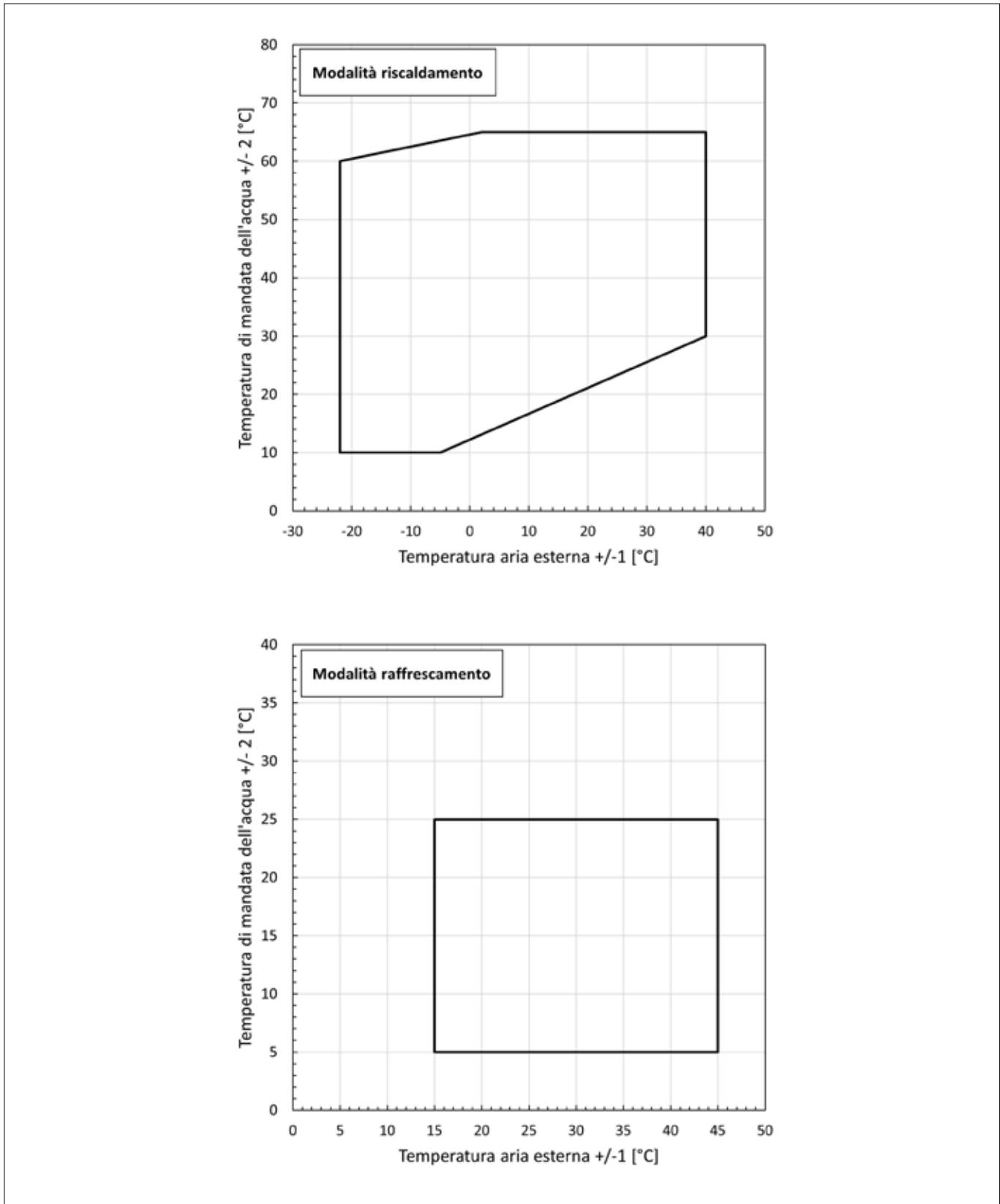
FIG. 8 (Modalità di riscaldamento e raffrescamento Serie SP - MP - LP - LP Plus)
