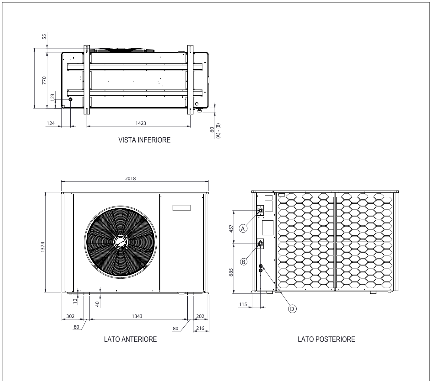
FIG. 5 (Dimensioni Serie L - LP Plus - LR Plus - con staffe)
