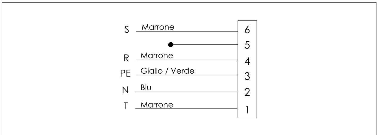
FIG. 84 (Cablaggio ventilatore)
