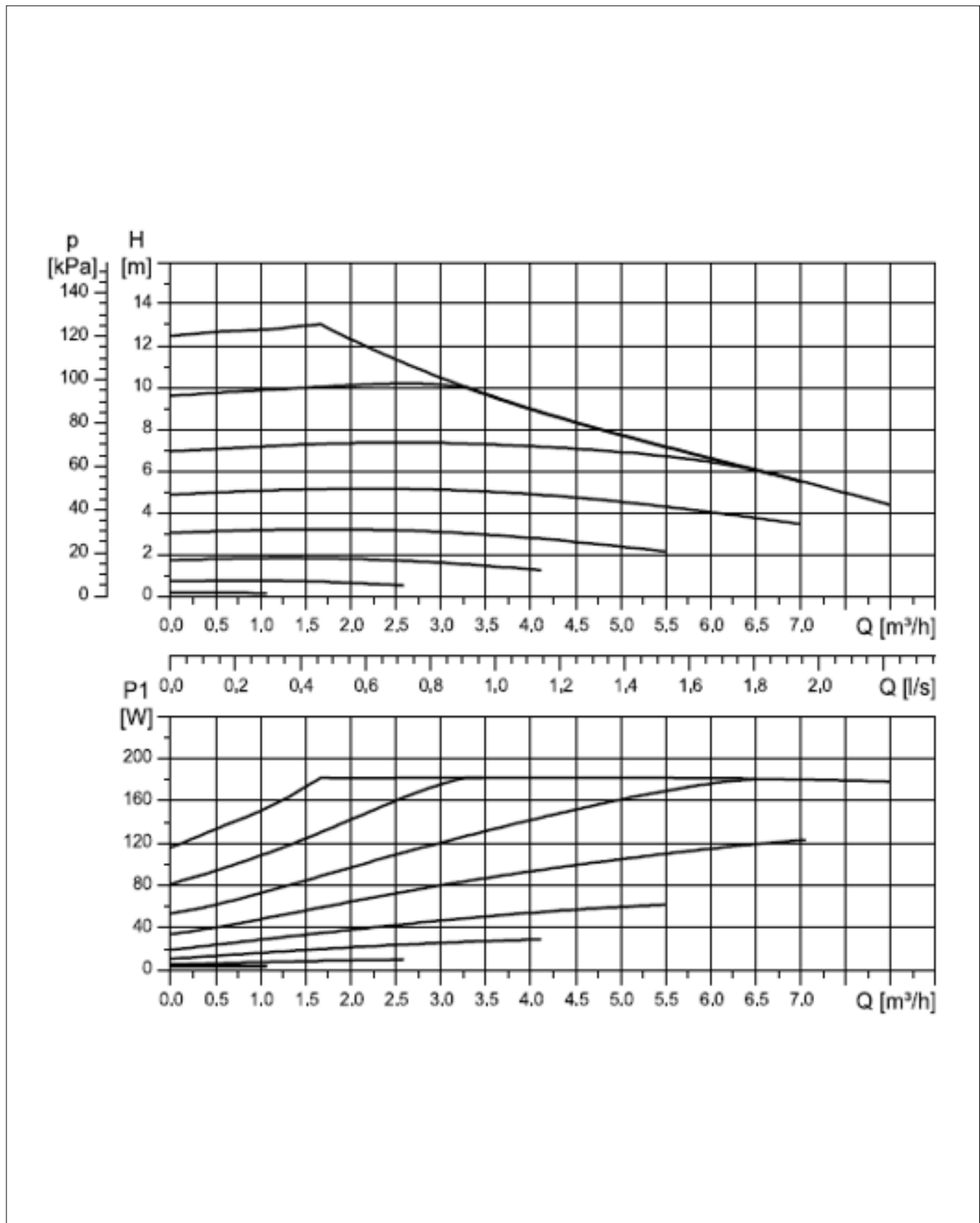
FIG. 18 (Curve e caratteristiche circolatore tipo Grundfos UPM10XL 25-125 180)
