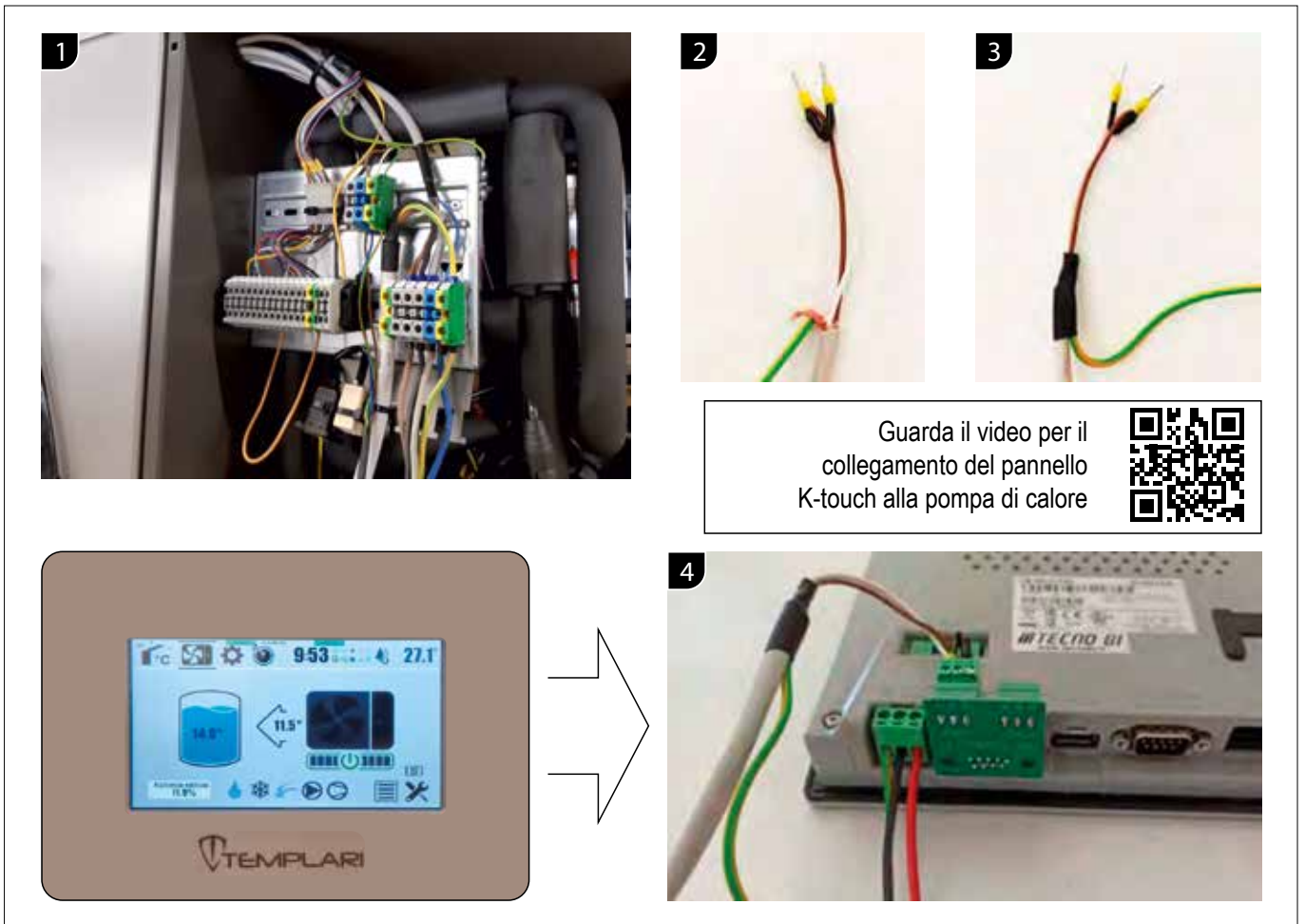
FIG. 67 (Connessione P-LAN 7a e connessione BMS 7b)
