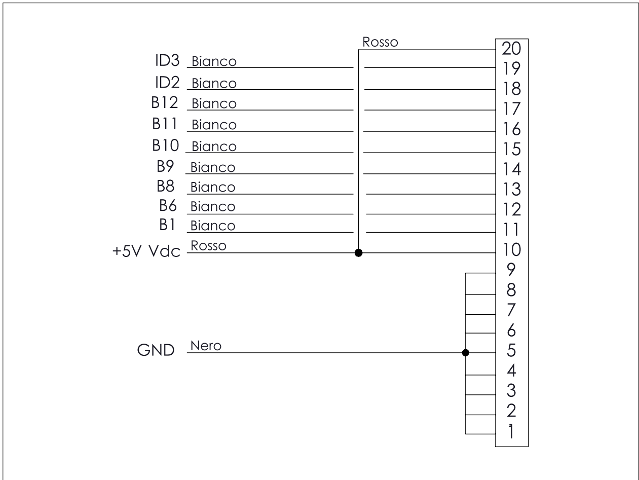
FIG. 86 (Cablaggio sonde)
