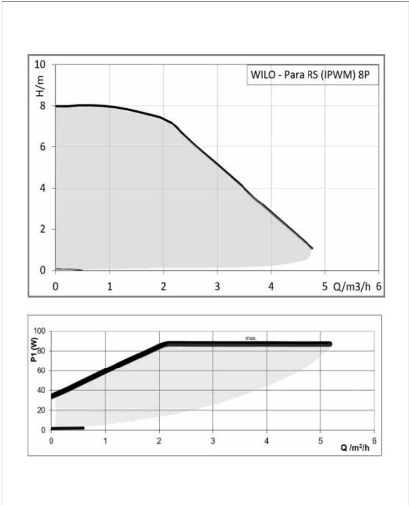
FIG. 12 (Curve e caratteristiche circolatore tipo Wilo Para 25/8 Plus e Wilo Para R 25/8 Plus)
