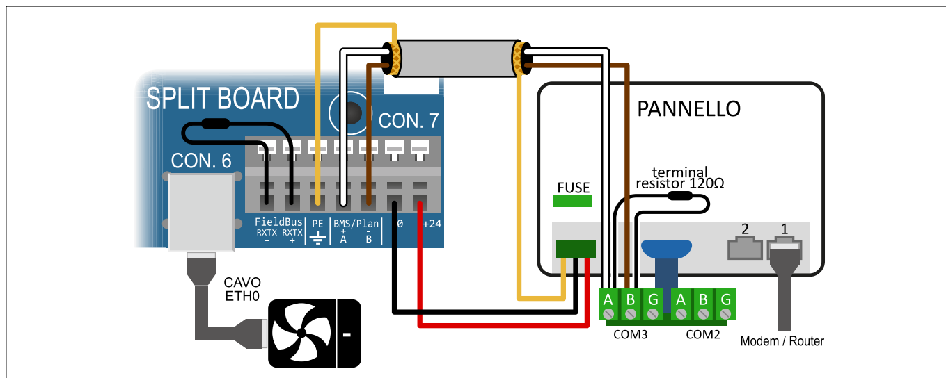
FIG. 65 (Collegamento K-Touch)
