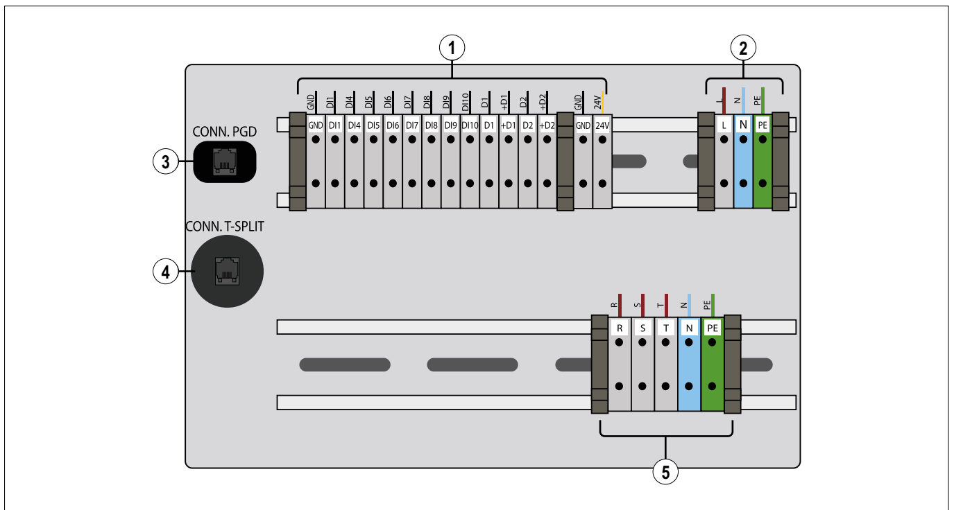
FIG. 50 (Morsettiera quadro elettrico secondario)
