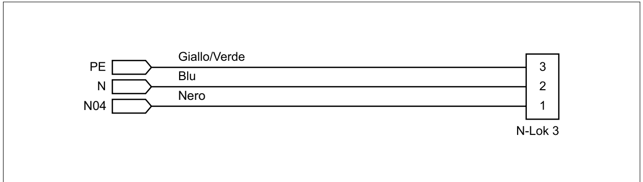
FIG. 83 (Cablaggio pompa di circolazione)
