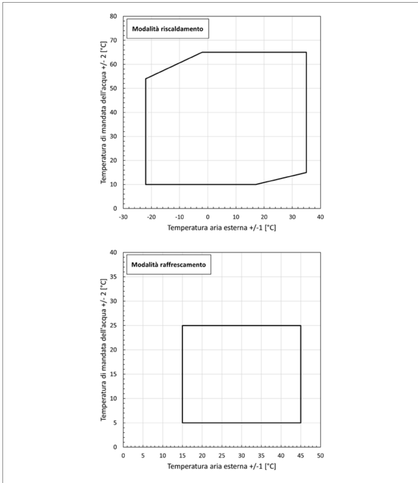
FIG. 6 (Modalità di riscaldamento e raffreddamento Serie SP-T)
