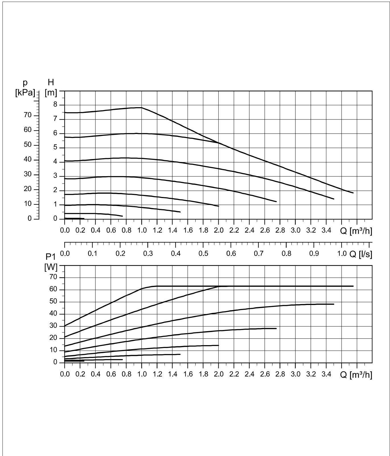
FIG. 20 (Curve e caratteristiche circolatore tipo Grundfos UPM4K 15-75 130 PWM)
