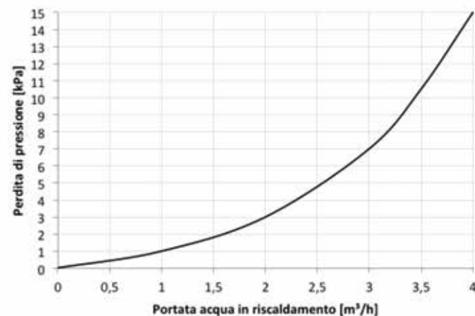
Perdita di pressione sullo scambiatore a piastre
