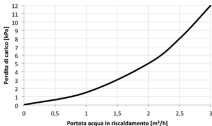
Perdita di carico sullo scambiatore a piastre
