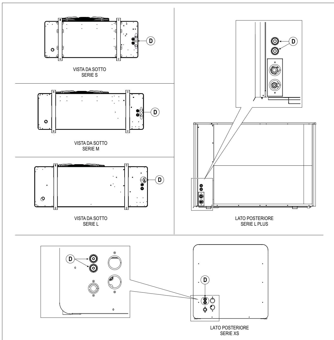
FIG. 42 (Collegamento alla fonte di energia elettrica)
