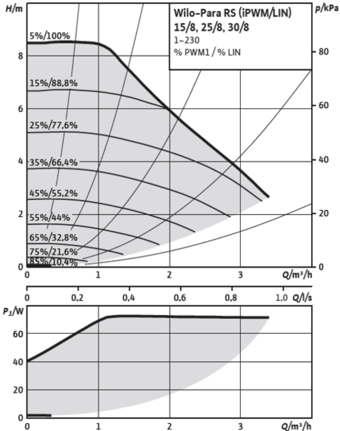
FIG. 10 (Curve e caratteristiche circolatore tipo Wilo Para 25/8 e Wilo Para R 25/8)
