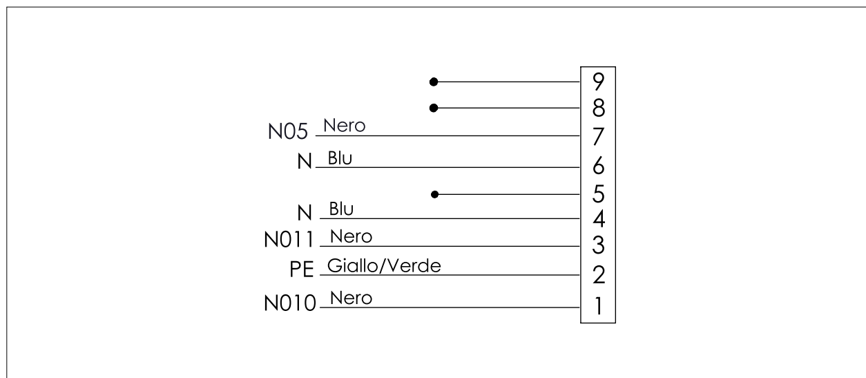
FIG. 81 (Cablaggio valvola 4 vie e resistenza carter)
