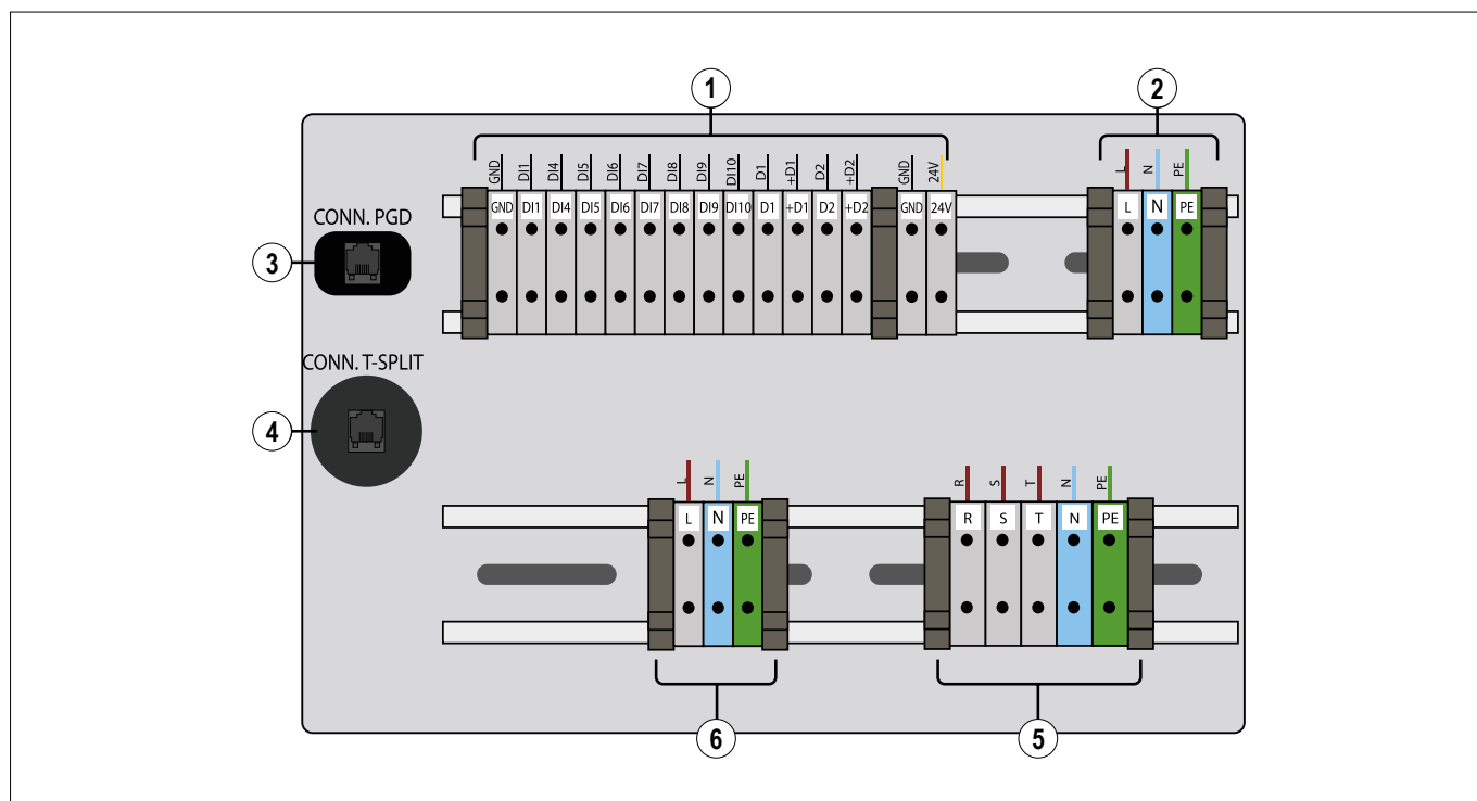
FIG. 47 (Morsettiera quadro elettrico secondario per PDC doppia alimentazione)
