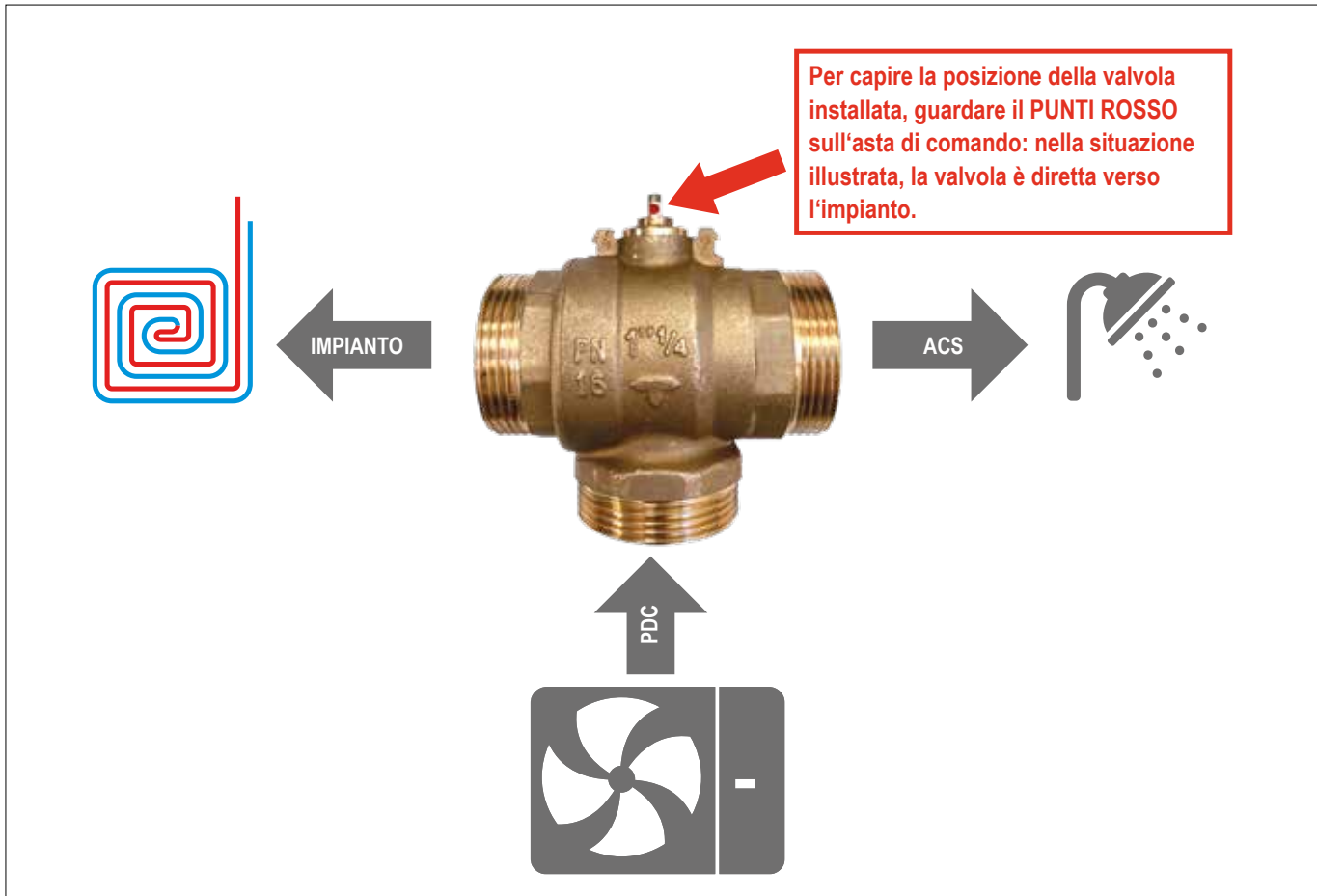
FIG. 51 (Collegamenti idraulici valvola a tre vie)
