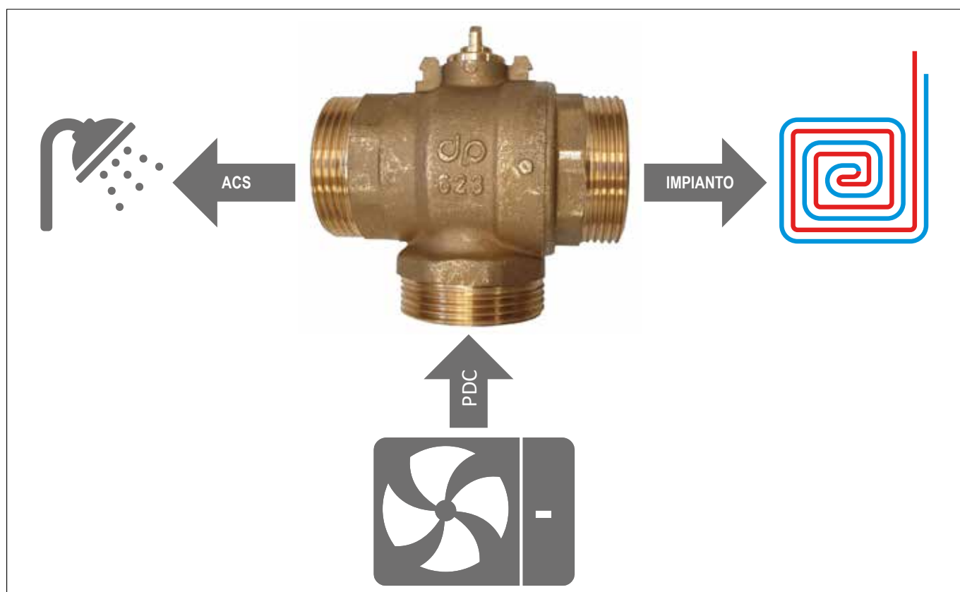
FIG. 50 (Collegamenti idraulici valvola a tre vie)
