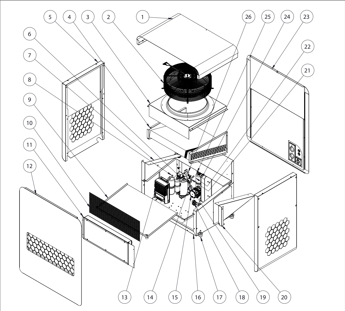
FIG. 22 (Denominazione dei componenti principali - Esempio modello XS versione Alta)
