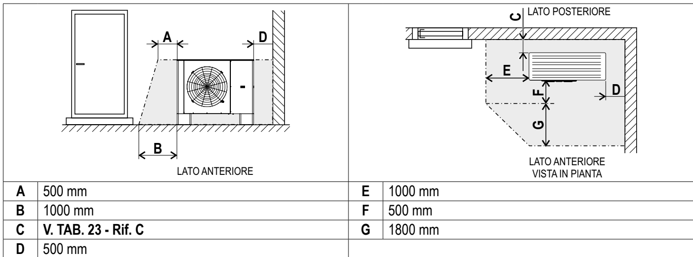
FIG. 32 (Zona di sicurezza in caso di installazione a terra in un angolo dell'edificio)
