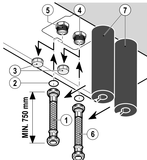
FIG. 37 (Collegamento alla fonte di energia idrica)
