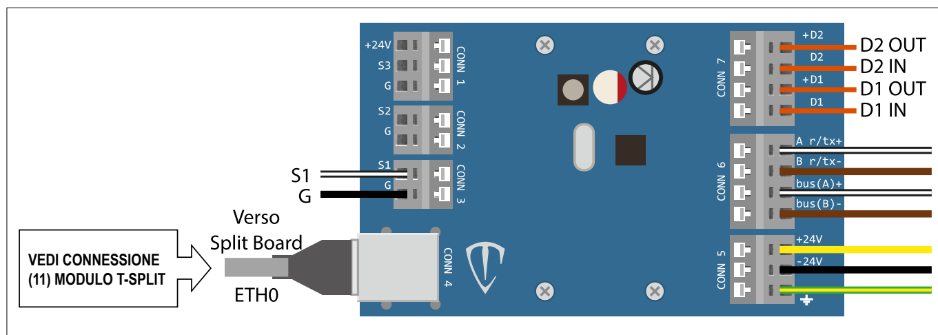
FIG. 56 (Scheda elettronica SG-Probe)
