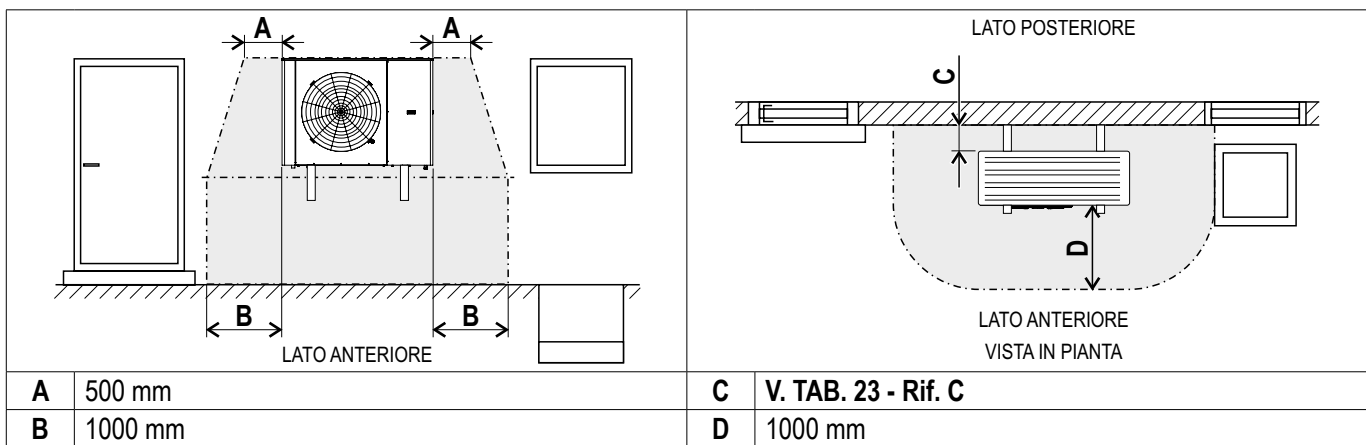
FIG. 33 (Zona di sicurezza in caso di installazione a parete davanti a una parete dell'edificio)
