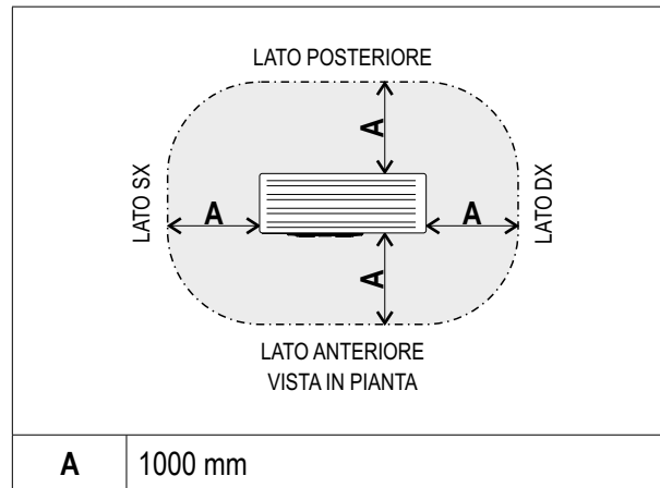
FIG. 30 (Zona di sicurezza in caso di installazione a terra - terreno o tetto piano)
