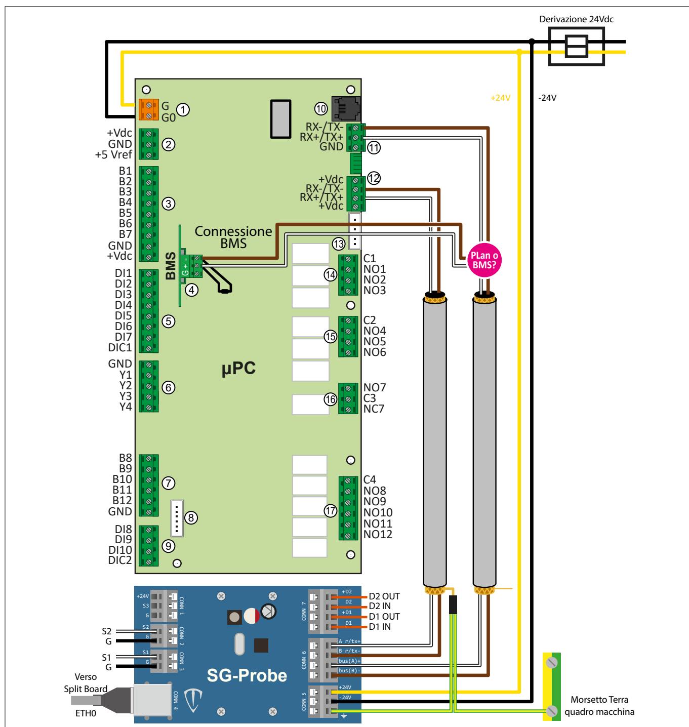
FIG. 43 (Cablaggio \mu PC unità esterna)
