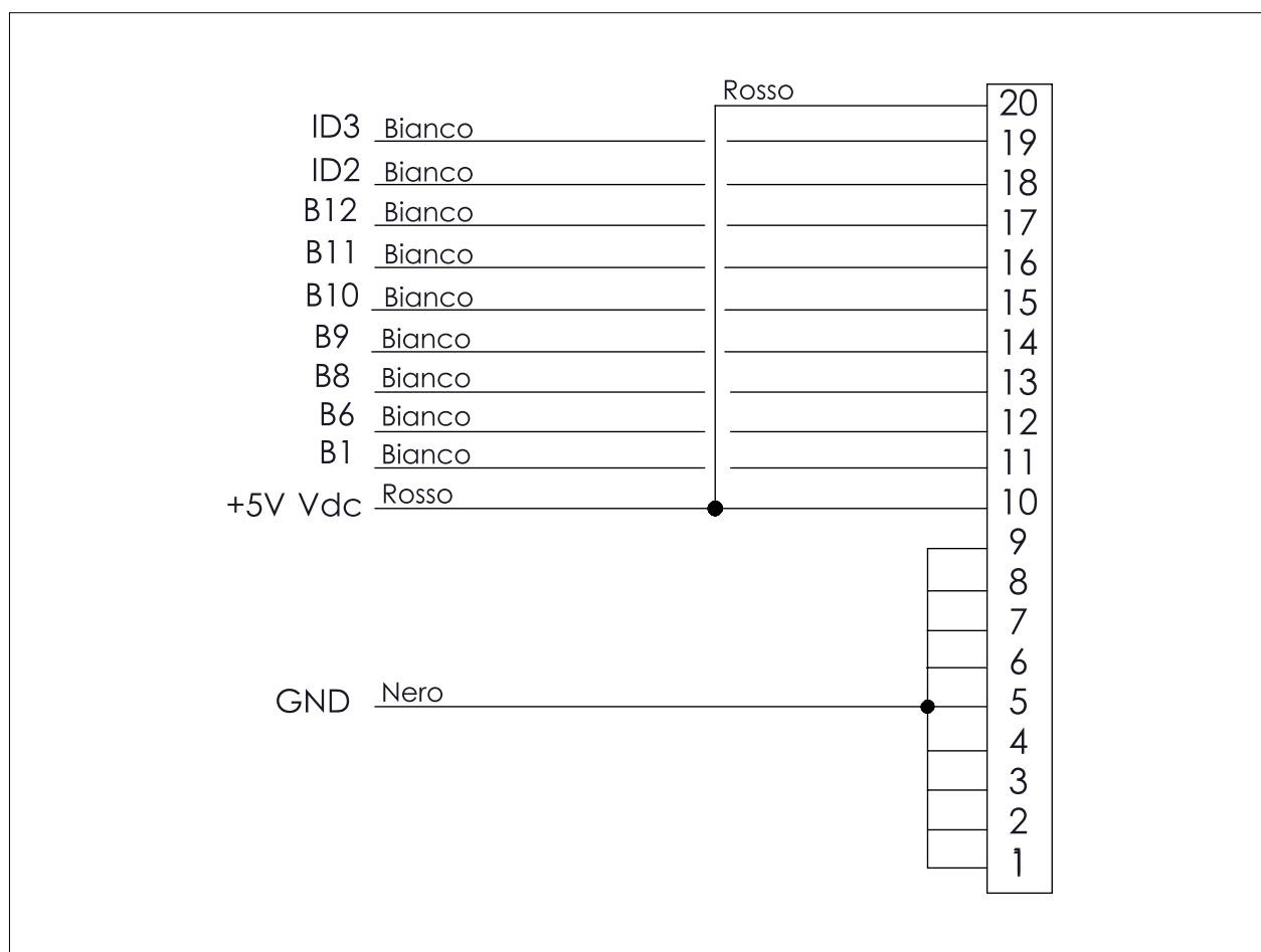
FIG. 82 (Cablaggio sonde)
