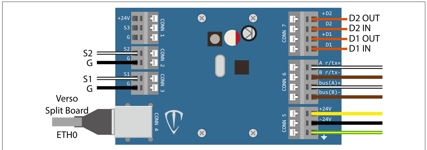
FIG. 45 (Scheda elettronica SG-Probe)
