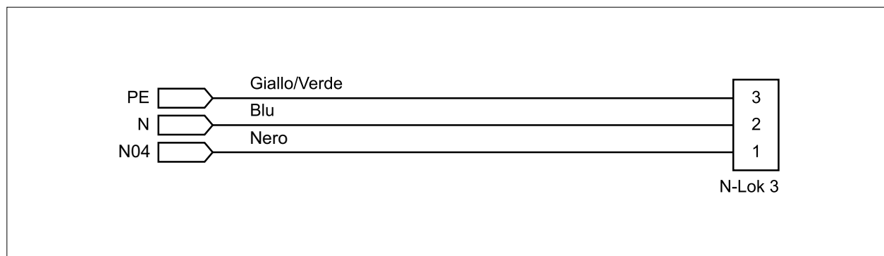
FIG. 79 (Cablaggio pompa di circolazione)
