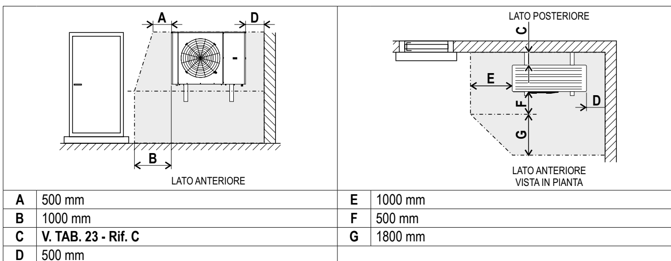
FIG. 34 (Zona di sicurezza in caso di installazione a parete in un angolo dell'edificio)
