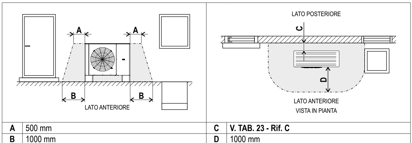
FIG. 31 (Zona di sicurezza in caso di installazione a terra davanti a una parete dell'edificio)
