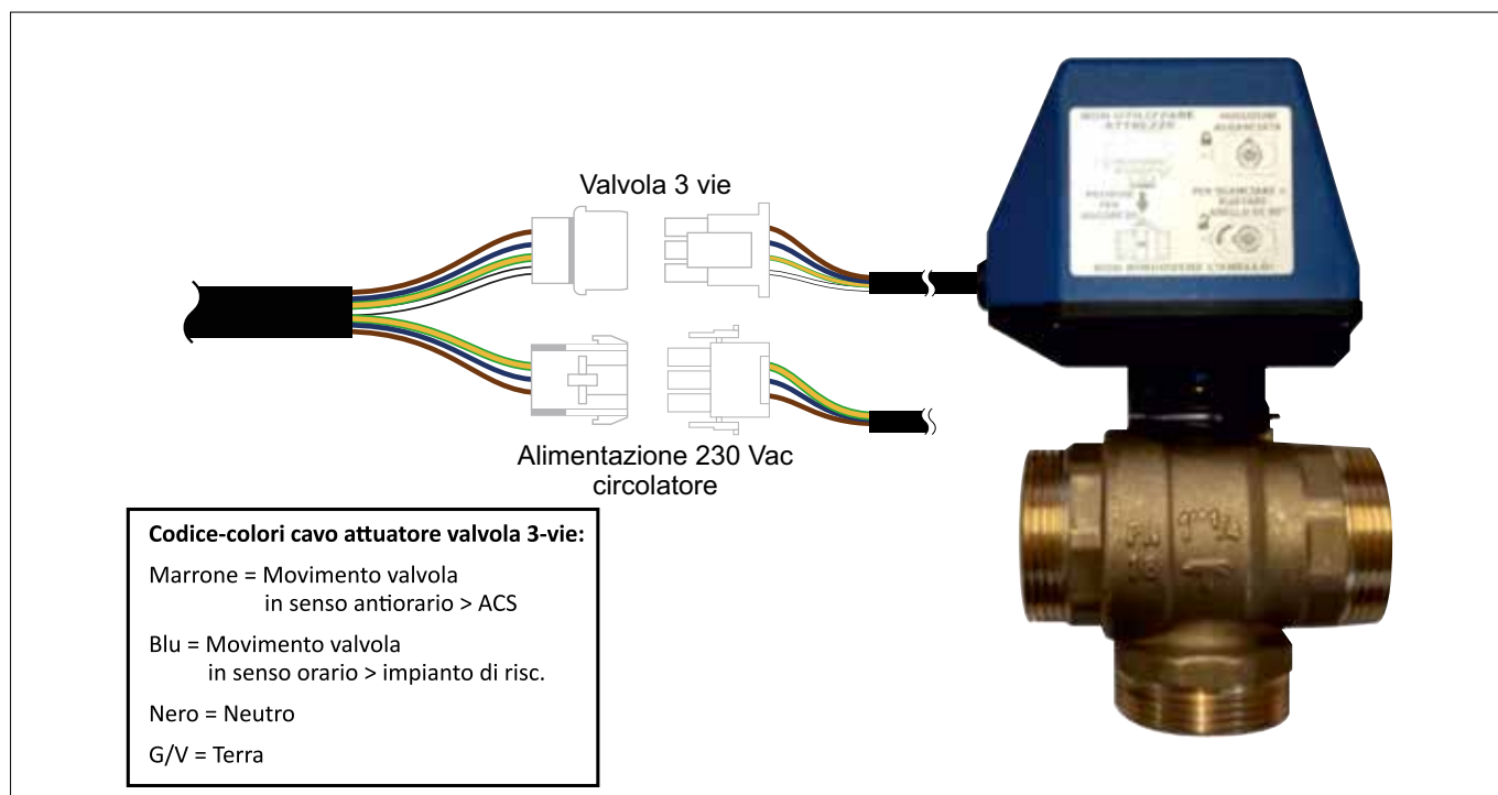
FIG. 49 (Collegamento valvola a tre vie)
